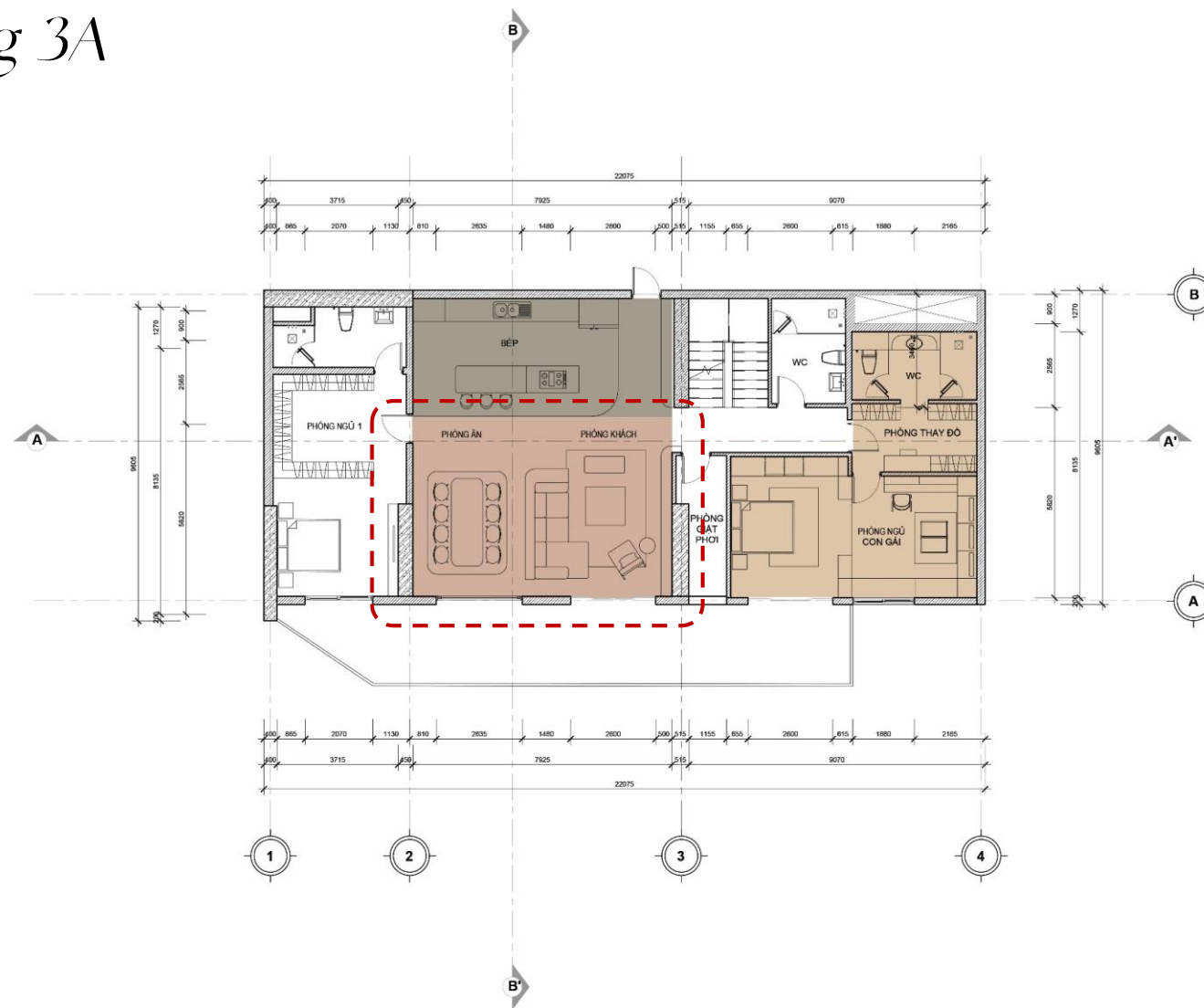
MẶT BẰNG TẦNG 3A
