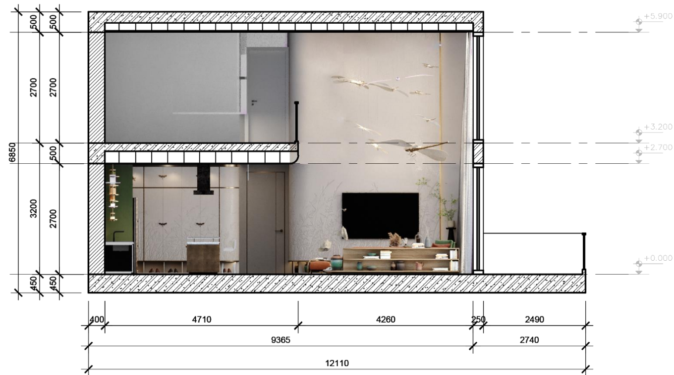
MẶT CẮT AA'
