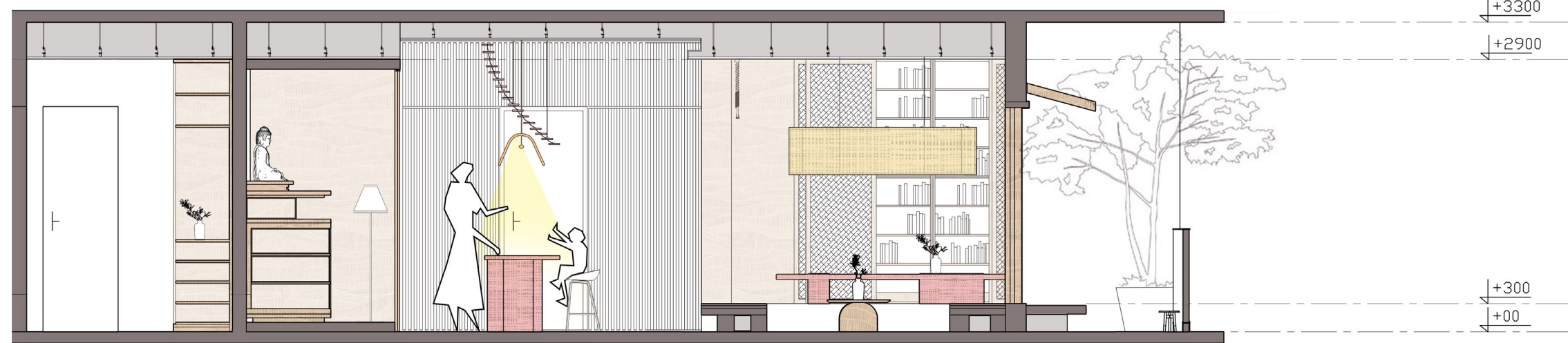
MẶT CẮT A-A
