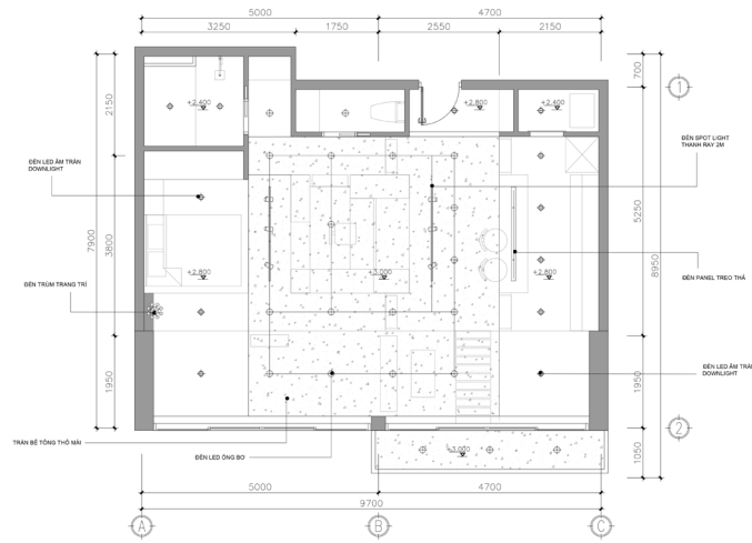
MẶT BẰNG BỐ TRÍ ĐÈN
