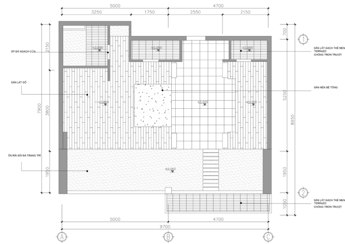
MẶT BẰNG SÀN
